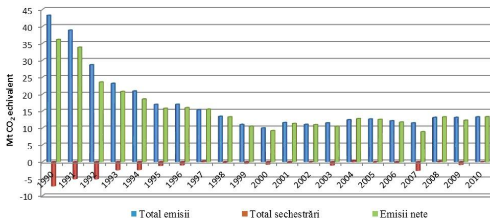
Figura 4. Dinamica emisiilor și sechestrărilor de gaze cu efect de seră în Republica Moldova, 1990-2010
